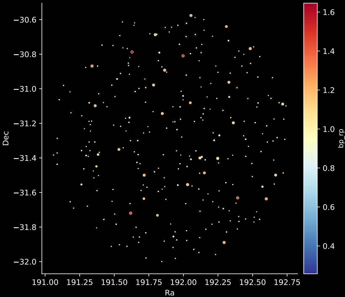
GALAH DR4 Field: [1779] Stars: 285
