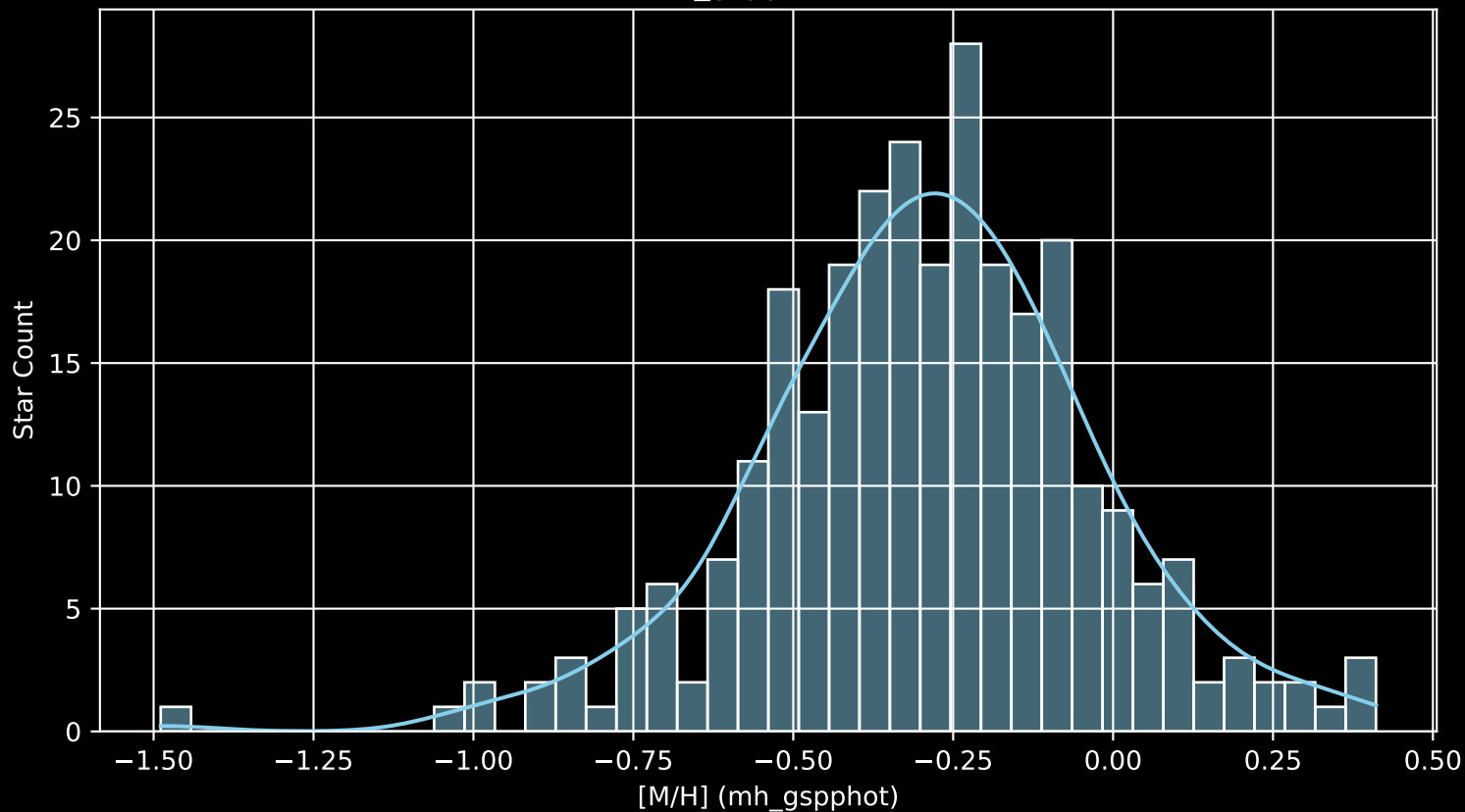
GALAH DR4 Field: [1779] [M/H] (mh_gspphot) (n= 285)
