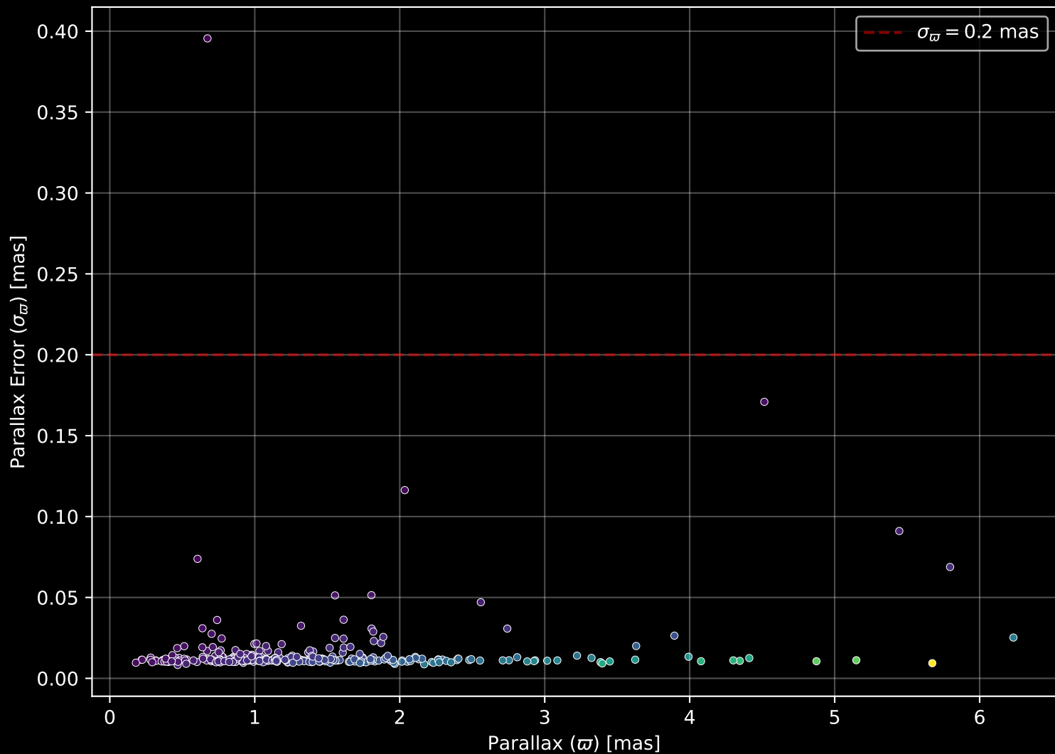
GALAH DR4 Field: [1779] Parallax Quality (n= 285)
