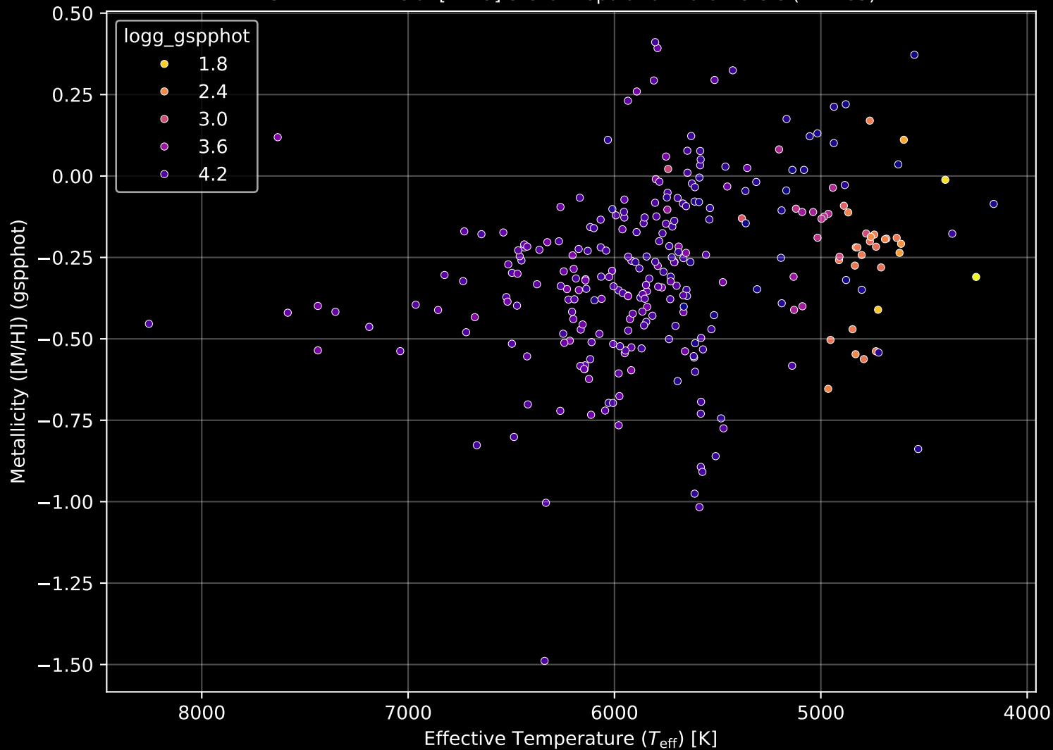
GALAH DR4 Field: [1779] Stellar Population Parameters (n= 285)
